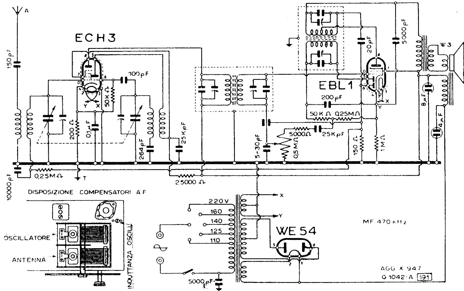
F.I.M.I. - MOD. PHONOLA « 301 »
